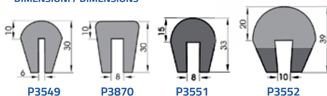
DIMENSIONI / DIMENSIONS
