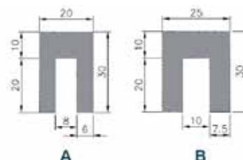
DIMENSIONI / DIMENSIONS
